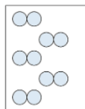
酸素
