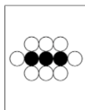
プロパン
