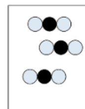
二酸化炭素
