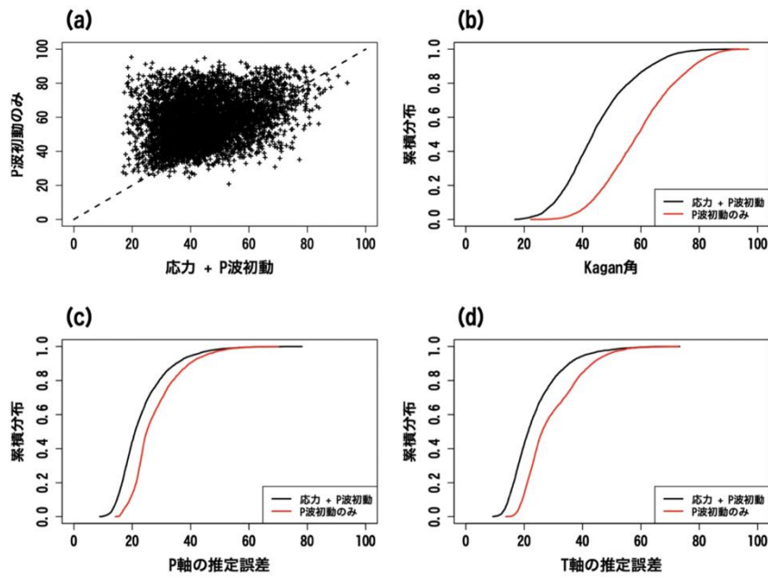
図2. 人工データを用いた2つのメカニズム解推定法の比較 (東北大学 [課題番号: 1206]) a) 両手法による結果を比較した散布図. 各々の地震に対する「応力情報あり」(応力+P波初動)と「応力情報なし」(P波初動のみ)の推定結果と真のメカニズム解からのズレを Kagan 角で表したもの. 値が大きいほどズレが大きい. 「なし」の推定結果のズレが「あり」のそれより大きい. b) Kagan 角の累積分布. この図でも全体として「なし」の Kagan 角の方が「あり」のそれより大きい. c) d) P 軸, T 軸の推定誤差. 「なし」の方が「あり」の場合より推定精度が低い.
