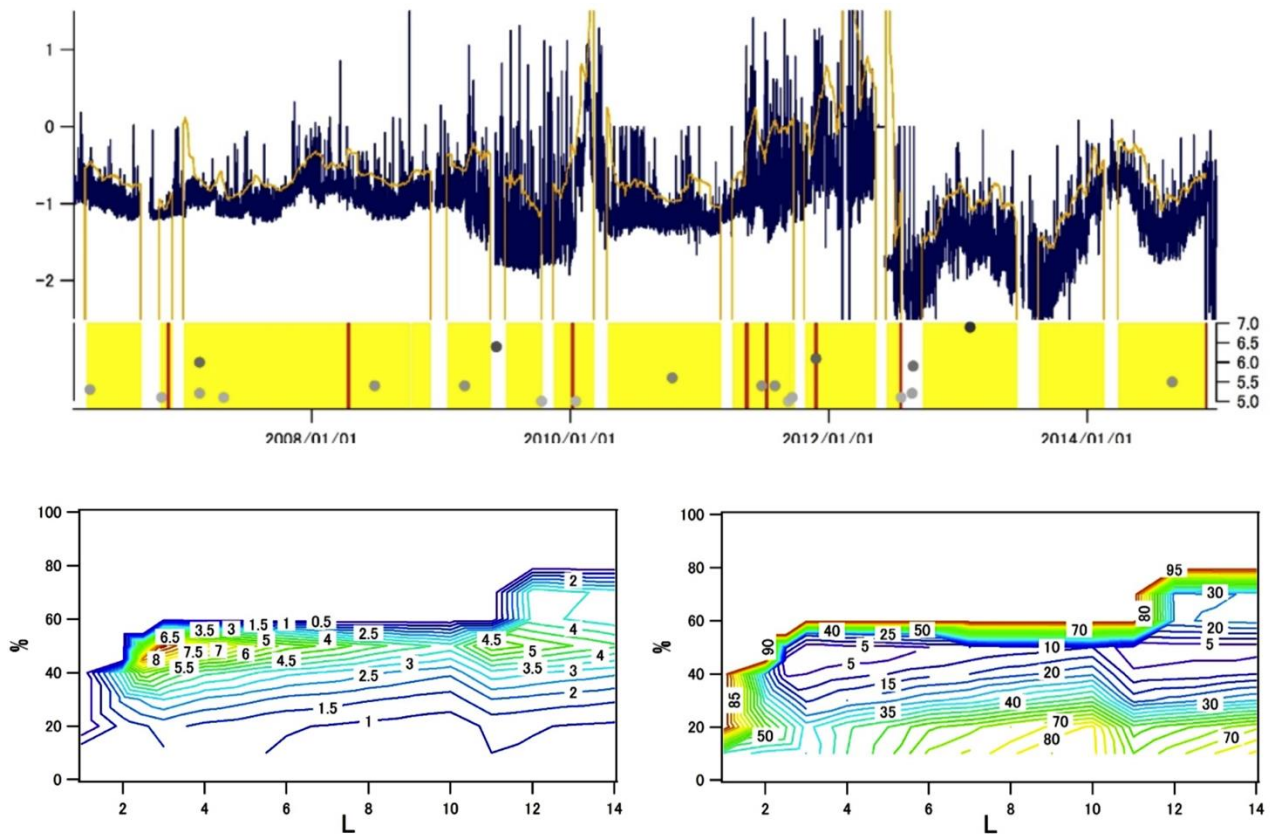
図18. VHF電波異常に基づく地震予測の検証（東海大学 [課題番号：2501]） (上)えりもでの広尾放送局の電波受信強度(紺)と、アダプティブに決めた閾値(オレンジ)の時系列。下の帯グラフが、黄色が警報OFF、赤色が警報ON期間をあらわす。帯グラフ上の丸が地震の発生した期間とそのときのマグニチュード(右軸)を示す。(左下)確率ゲインの等高線図。異常と判断するための検出時間割合の閾値(縦軸)と警報持続時間をチューニングパラメタとした。(右下)p値(%)の等高線図。縦軸、横軸は左下と同じ。
