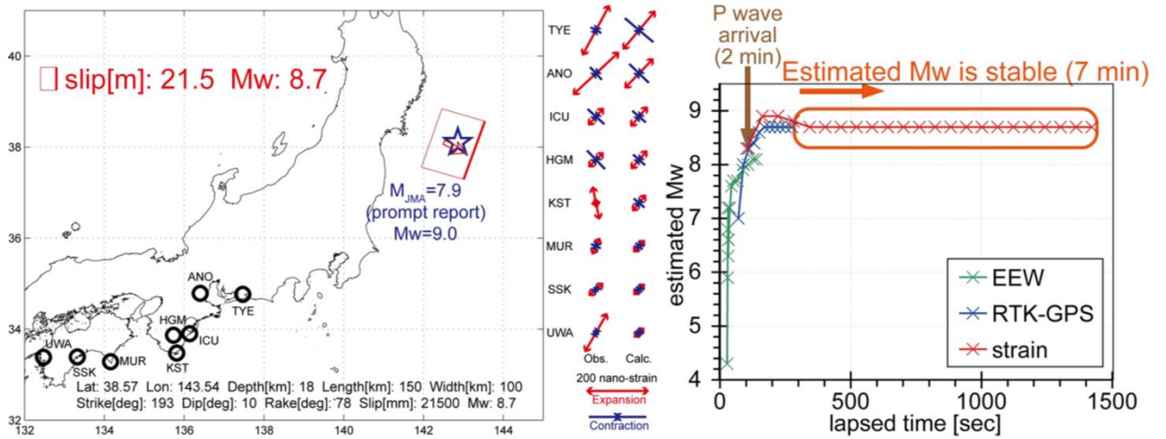
図9. ボアホールひずみ計による巨大地震のモーメントマグニチュードの即時推定 (Itaba, 2018, 産業技術総合研究所 [課題番号: 5007])
