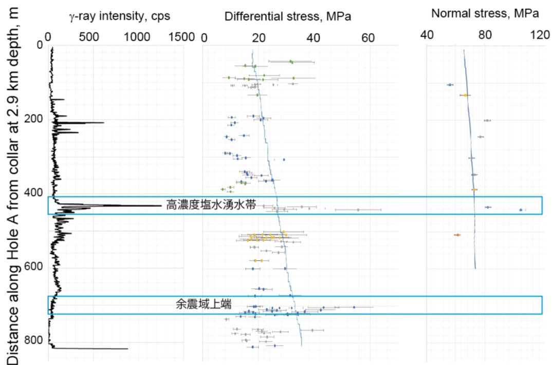
図4. ICDP-DSeisで掘削されたHoleAの解析結果（東北大学流体研究所〔課題番号：2948〕） 左から順に、孔内検層による自然ガンマ線強度、DCDAにより測定された孔井直交面内の差 応力、DRAにより測定された孔軸方向の法線応力の深さ分布応力分布に記された青実線は、 弾性数値モデルから期待される応力値. 400m地点では、高濃度塩水の湧出がみられた. Hole Aは余震域に交差していないが、700m地点で余震発生深度に達している.
