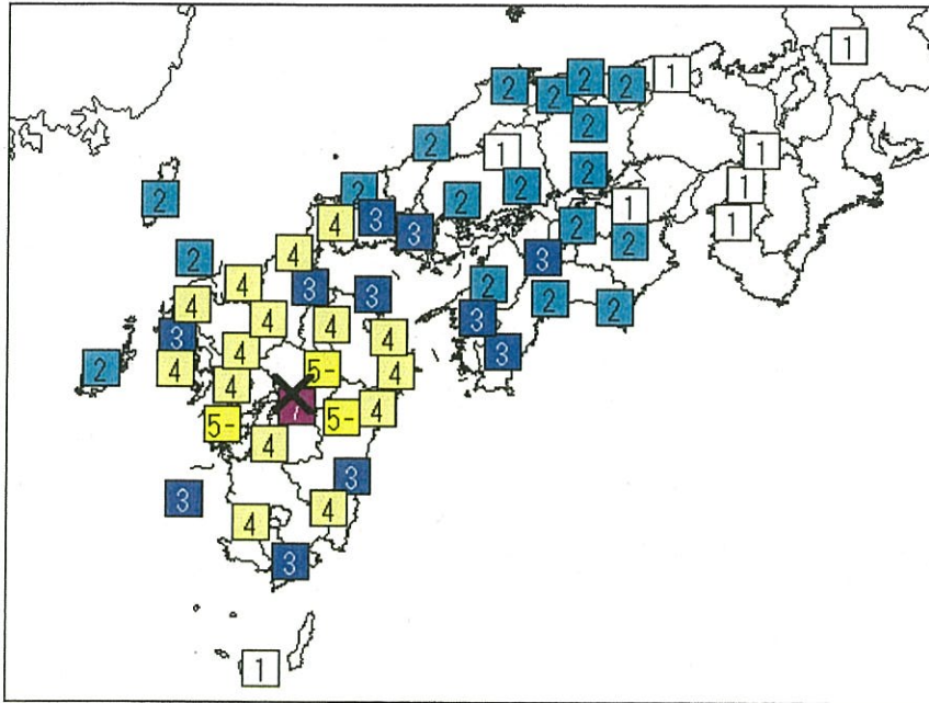
各地域の震度分布
