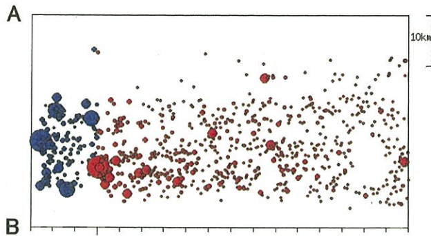
震央分布図の四角形領域内の地震活動経過図
