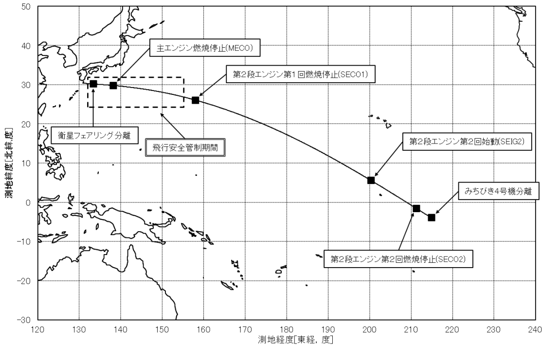
H-IIA/F36 シーケンス・オブ・イベント
