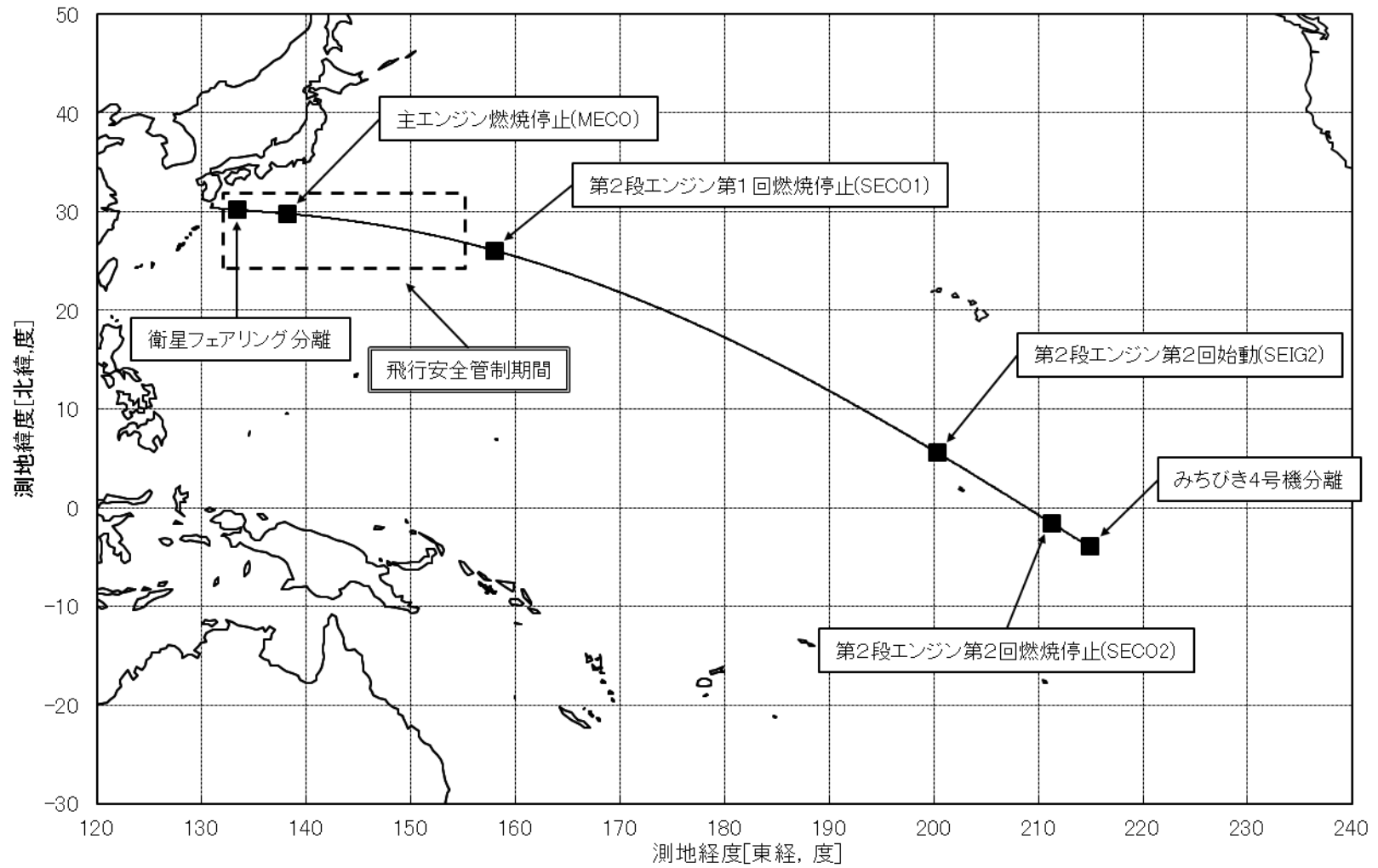
図1 H-IIAロケット36号機の飛行経路概要(機体現在位置)
